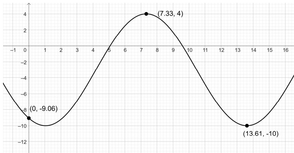
Figura 1: Gráfico de una función periódica del tipo f(x) = A \sin(Bx + C) + D .
